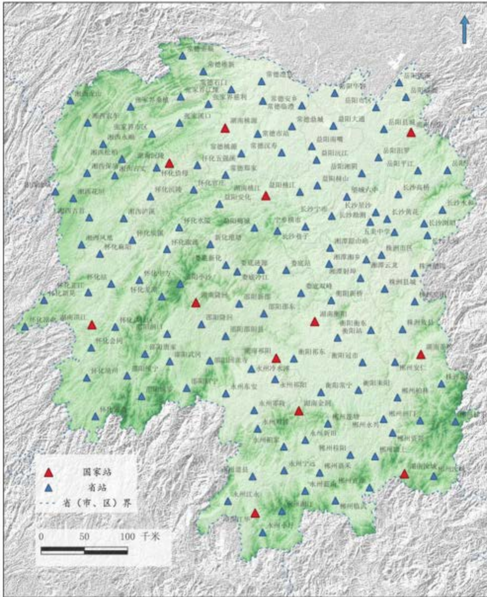
图 1-3 湖南省北斗卫星导航定位基准站网（HNCORS）分布图
