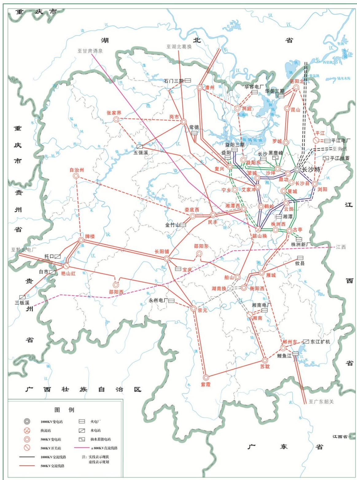
图8 湖南省“十四五”500千伏及以上电力系统规划接线图
